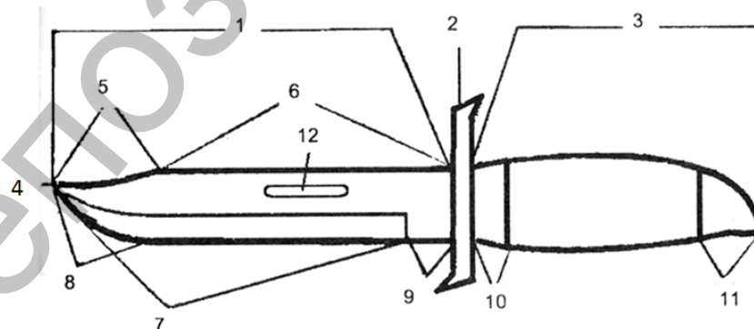
НОЖ: 1 – клинок, 2 – упор, 3 – рукоять, 4 – острие, 5 – скос обуха, 6 – обух, 7 – лезвие, 8 – закругление лезвия, 9 – пятка клинка, 10 – кольцо, 11 – наконечник, 12 – дола.
