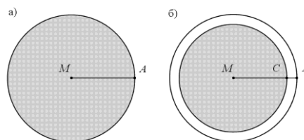
Рис. 3. Вид электродов терморезисторов (а – классический вариант, б – модифицированный терморезистор).
