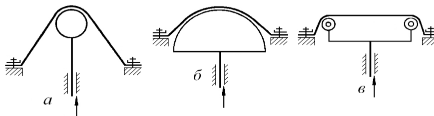
Рис. 1. Схемы нагружения материала при двухосном растяжении.
