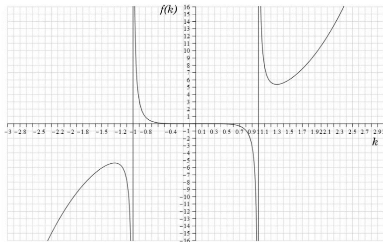
Рисунок 2 – График функции f(k) = \frac{k^5}{k^2-1}
