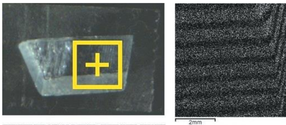
Рисунок 2 – Карты распределения хрома в образце TGS – TGS + Cr по данным рентгенофлуоресцентного анализа (РФЛА: a – спектрометр XGT-7200)
