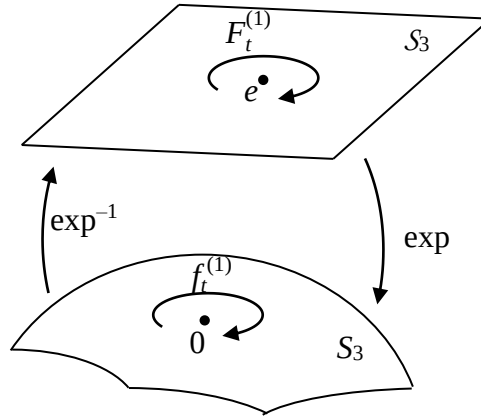
Рис. 3. Построение однопараметрической группы подобий
