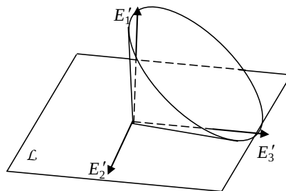
Рис. 2. Расположение базисных векторов
