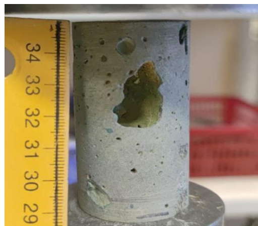
Рисунок 2 – Крупная пора в боковой поверхности керна базальта
