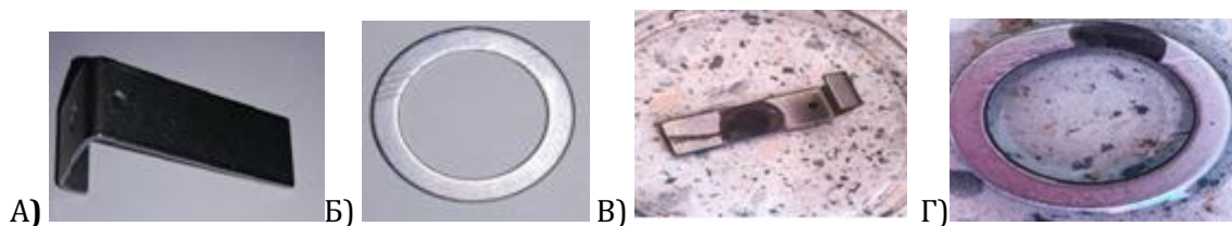
Рисунок – Детали до (А, Б) и после (В, Г) нанесения раствора, для удаления цинкового покрытия
