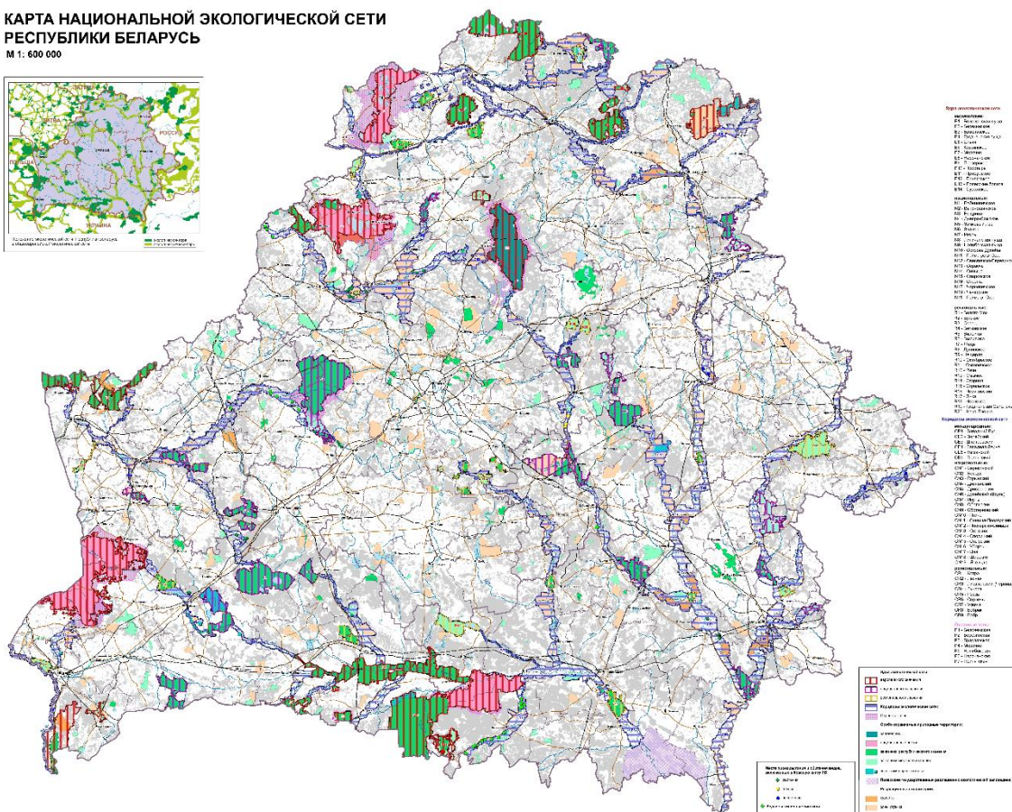
Рисунок 1 – Схема Национальной экосети Республики Беларусь
