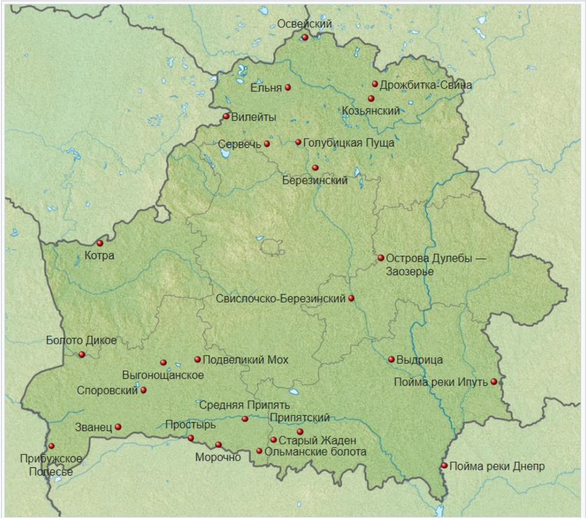
Рисунок 3 – Карта Рамсарских угодий
