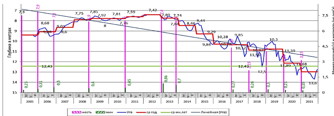
Рисунок 1 – Совмещенный график колебания среднегомесячного уровня (м), минерализации (г/л), и общей жёсткости (мг-экв/л) ПВ по скв. 419 Кошрабатского месторождения
