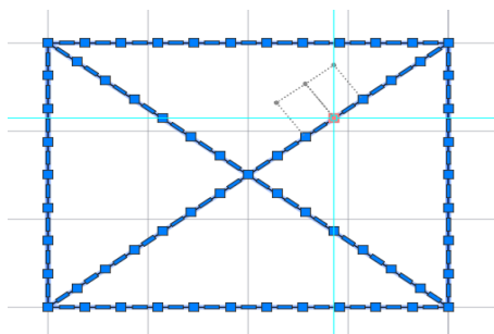
Рисунок 5 – Контур закрепки с координатами узлов
