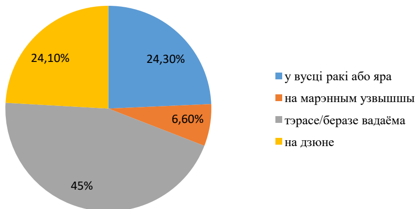
Статыстыка тапаграфічнага размяшчэння стаянак познеледавіковага часу на тэрыторыі Беларусі
