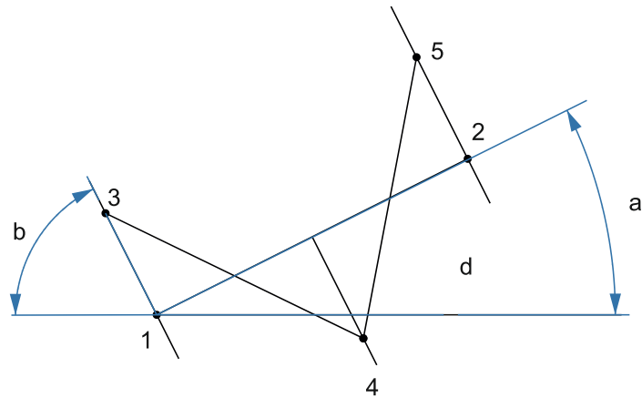
Рисунок 3 – Расчетная схема
