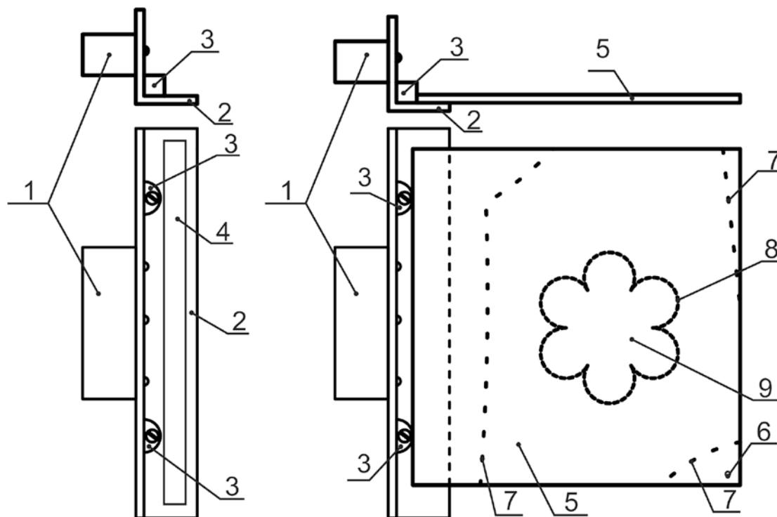
Рисунок 2 – Последовательность изготовления оснастки
