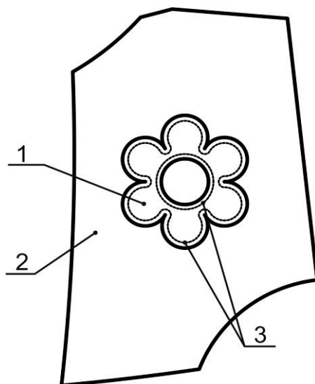
Рисунок 1 – Конструкция настрачиваемой аппликации
