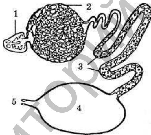
Рис.5.3. Выделительная система речного рака (антеннальная железа): 1 - целомический мешочек; 2- лабиринт; 3 – почечный канал; 4 - мочевого пузыря; 5 - выделительная пора.
