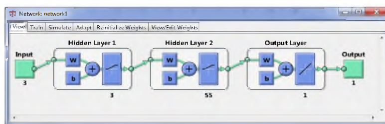
Рисунок 1 – Окно моделирования нейронной сети View
