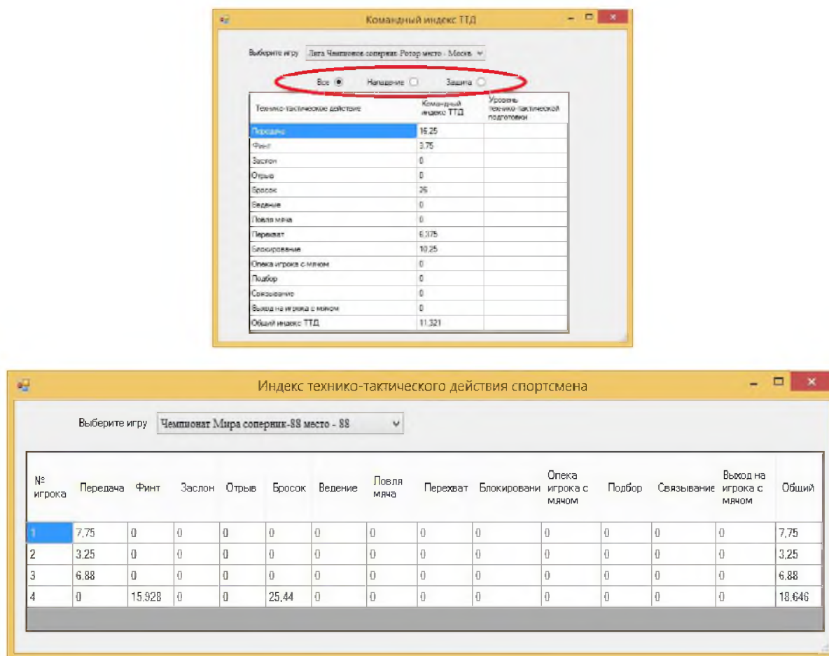
Рисунок 4 – структура разделов «Командный индекс ТТД» и «Индекс ТТД спортсмена»
