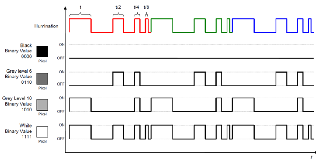
Рисунок 1 – Пример использования временного метода синтеза изображения с оттенками серого.
