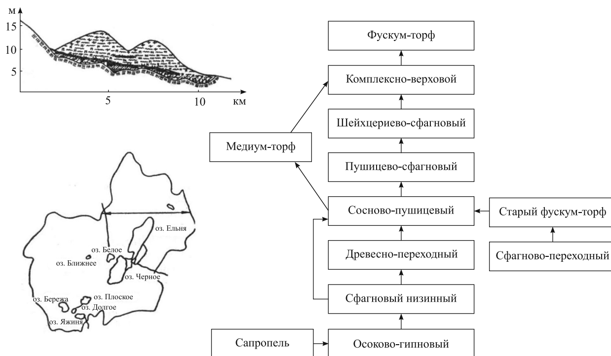
Рис. 2. Структура торфяной залежи болотного массива Елья [7]
