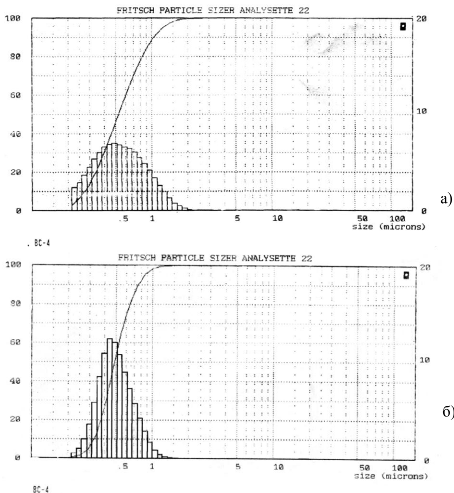
Рисунок 1 Результаты гранулометрического анализа а) исходный порошок; б) активированный порошок
