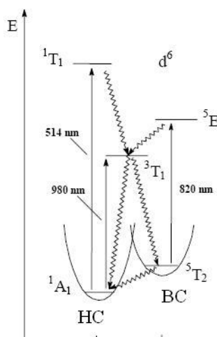
Рисунок.1. Диаграмма переходов при фотовозбуждении для [\text{Fe}(\text{ptz})_6](\text{BF}_4)_2
