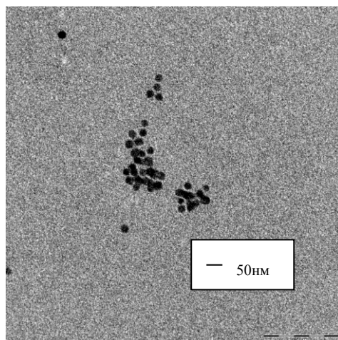
Рис. 1. Электронная микрофотография наночастиц золота
