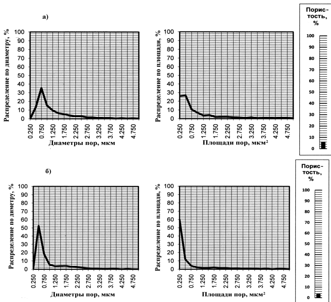
Рис. 2 – Распределение пор по диаметру и по площади в керамических материалах, полученных из обычных (а) и активированных ультразвуком порошков (б)
