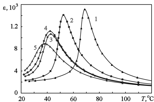
Рис. 2 – Температурные зависимости диэлектрической проницаемости керамики \text{Ba}_{0.8}\text{Sr}_{0.2}\text{TiO}_3:\text{Mg} при различной концентрации магния: 1- 0; 2 - 0.5; 3 - 1.0; 4 - 1.5; 5 - 2.0 мол. %
