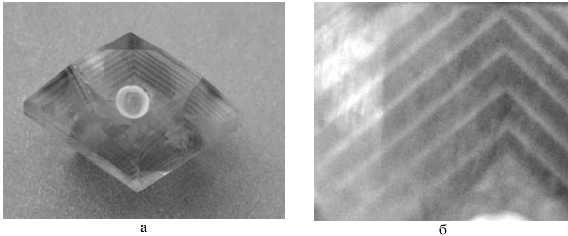
Рисунок 1 – Внешний вид кристалла ТГС-ТГС:Cr +3 (а) и его увеличенный фрагмент (б)
