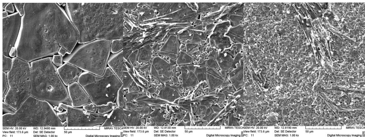
Рис. 1 – Микроструктура керамики Ba_{0.8}Sr_{0.2}TiO_3:Mg : содержание магния а) - 0, б)- 0.5, в)-1.0.
