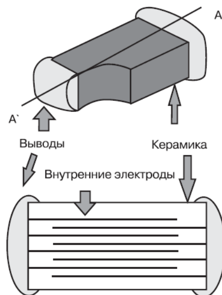
Рис. 1 – Схематичное изображение многослойного конденсатора
