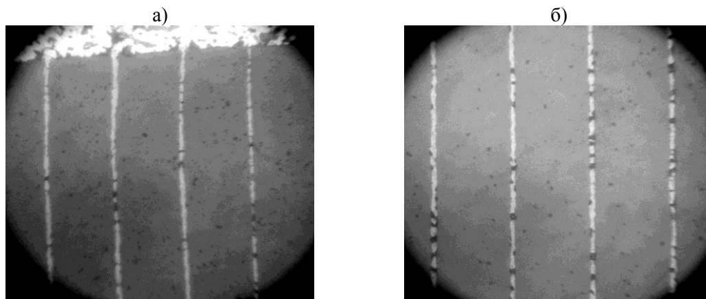
Рис.1 – Микрофотографии шлифов многослойных конденсаторов, полученных из обычных (а) и активированных ультразвуком порошков (б)
