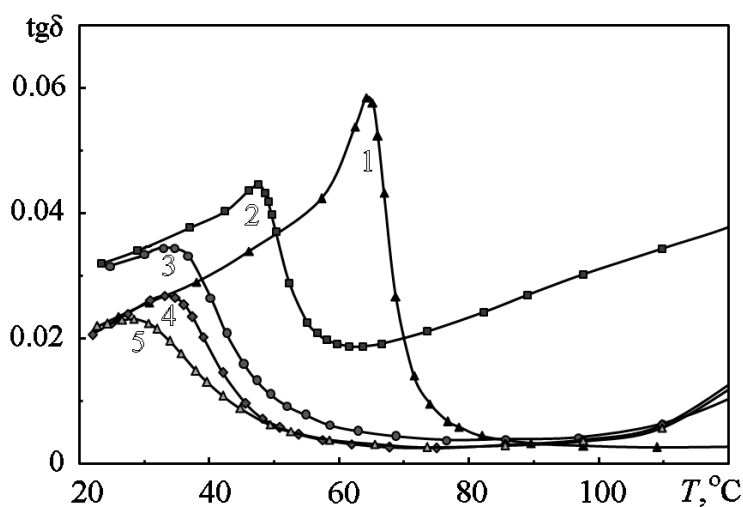
Рис. 3 – Температурные зависимости тангенса угла диэлектрических потерь керамики \text{Ba}_{0.8}\text{Sr}_{0.2}\text{TiO}_3:\text{Mg} при различной концентрации магния: 1 - 0; 2 - 0.5; 3 - 1.0; 4 - 1.5; 5 - 2.0 мол. %
