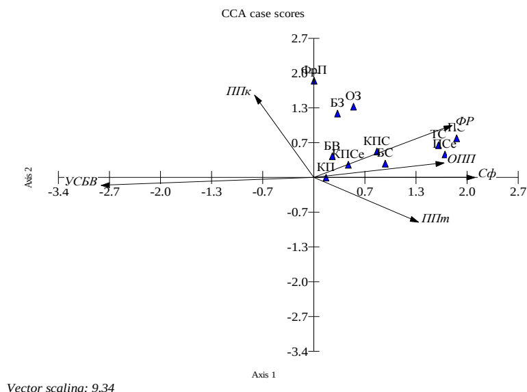
Рисунок 1. – Диаграмма ординации ССА-взаимосвязи факторов среды и энтомокомплексов (Insecta:Auchenorrhyncha, Heteroptera, Coleoptera) сообществ растений различной степени трансформации
