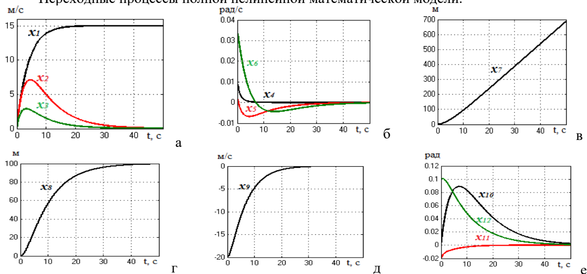
Рисунок 2 – Переходные процессы
