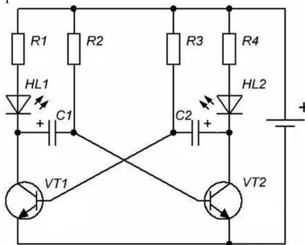
Рисунок 1 – Схема мультивибратора
