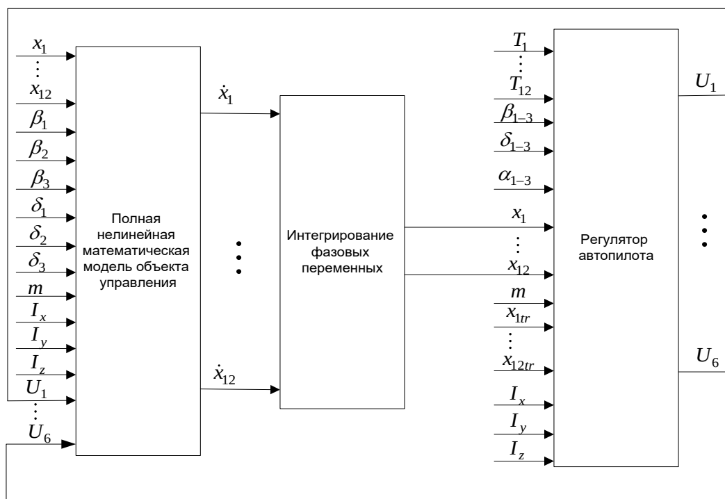
Рисунок 1 – Модель пространственного движения ЗУР
