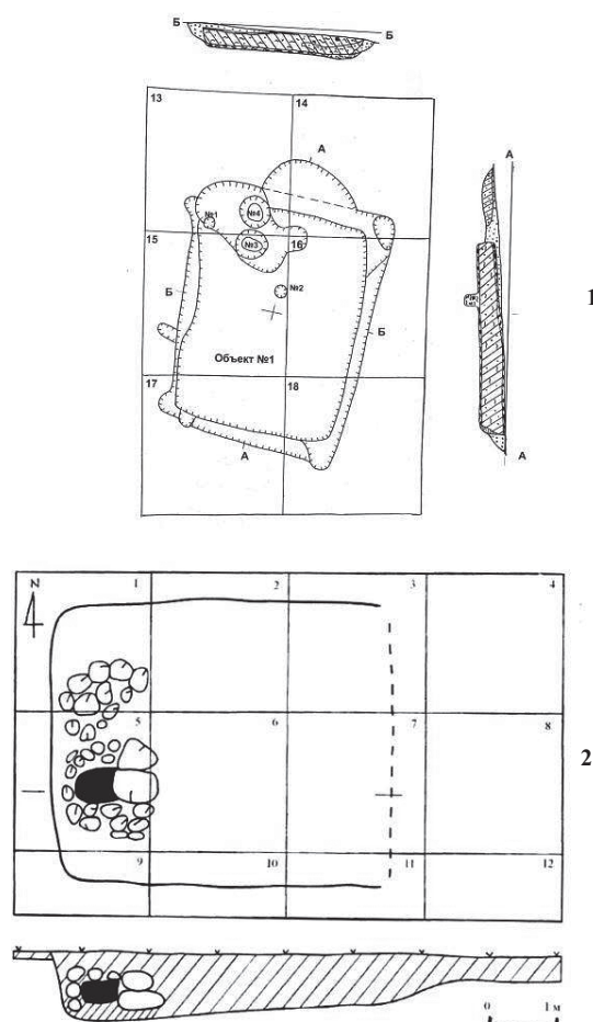
Рис. 4. Типы построек середины – третьей четверти I тыс. н.э. на селищах Зарово (1) и Лужесно (2) Витебского района
