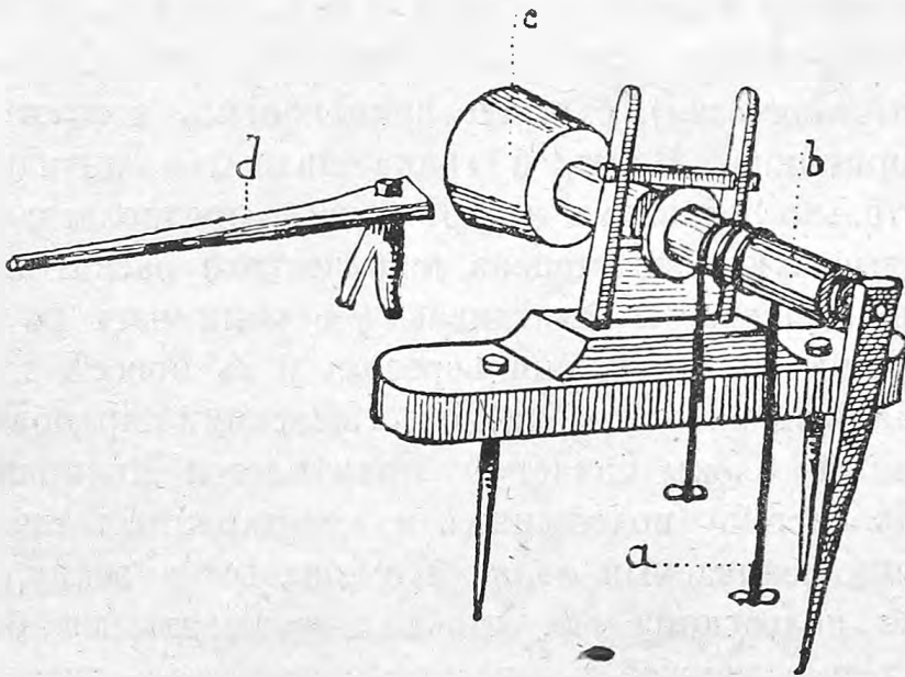
Фиг. 57.—Калмыцкій токарный станокъ съ поперемяннымъ вращательнымъ движеніемъ, получающимся съ помощью веревки (а), намотанной въ нѣсколько оборотовъ на ось (b); (c)—деревянный чурбанъ, изъ котораго предполагается выточить чашку; (d)—скамья для токаря. (По Reuleaux).
