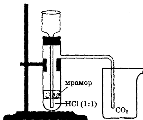
Рисунок 4 — Получение оксида углерода(IV)
