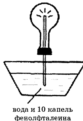
Рисунок 2 — Растворимость аммиака
