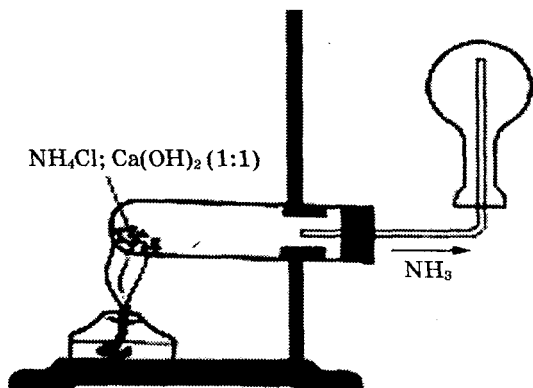
Рисунок 1 — Получение аммиака
