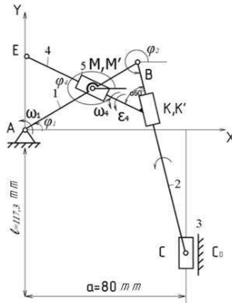
Рис. 3. Кинематическая схема
