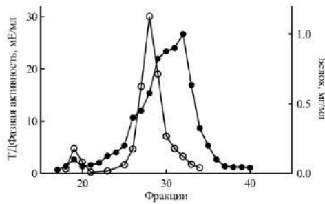
Рис. 3. Хроматография экстракта из печени курицы на колонке с тойоперлом HW-55, ● – концентрация белка, ○ – ферментативная активность при pH 9,0
