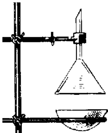
Рис. 15. Прибор для получения P_2O_5
