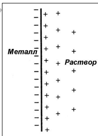
Рис. 7. Двойной электрический слой на границе раздела металл-раствор
