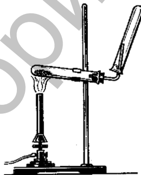
Рис. 14. Прибор для получения аммиака
