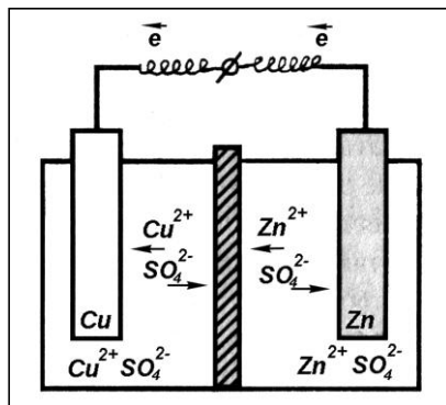
Рис. 6. Схема медно-цинкового гальванического элемента
