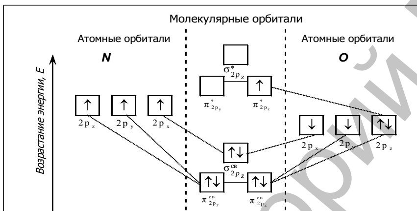
Рис. 5. Энергетическая схема заполнения электронами молекулярных орбиталей в молекуле NO (показаны только 2p -электроны)
