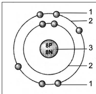
Рис. 1. Планетарная модель строения атома кислорода. (пояснения см. в тексте)
