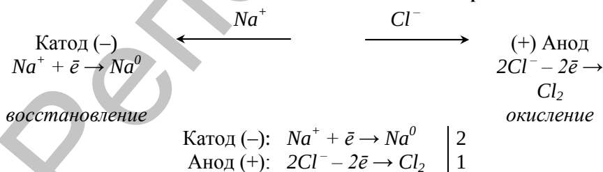
Рис. 8. Схема установки для электролиза NaCl
