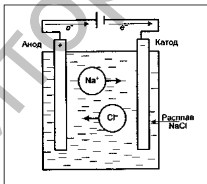
Рис. 8. Схема установки для электролиза NaCl
