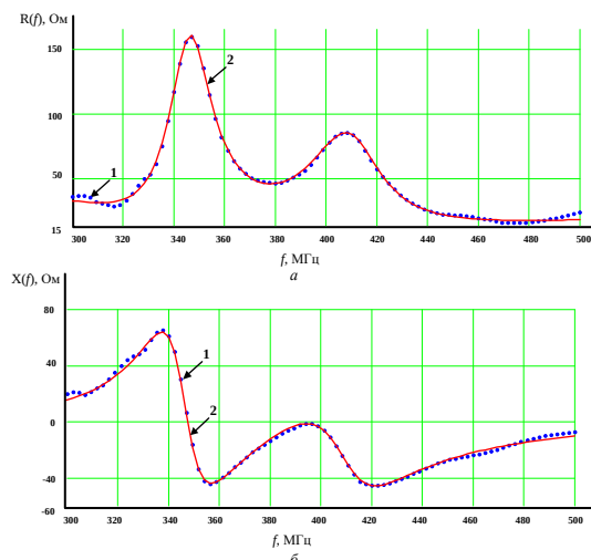
Рисунок 1 – Зависимость изменения активной (а) и реактивной (б) части импеданса АУ AD-25/CW-3512 в рабочей полосе частот ( \Delta f = 200 МГц): 1 – значения, измеренные в помещении; 2 – аппроксимированные значения.
