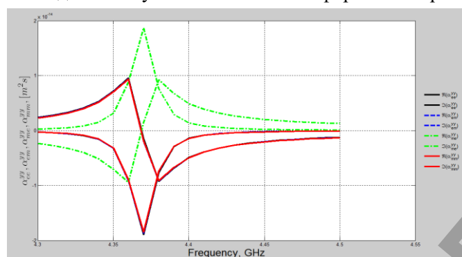
Рисунок 3 – Графики частотной зависимости действительной и мнимой частей поляримостей планарной спирали
