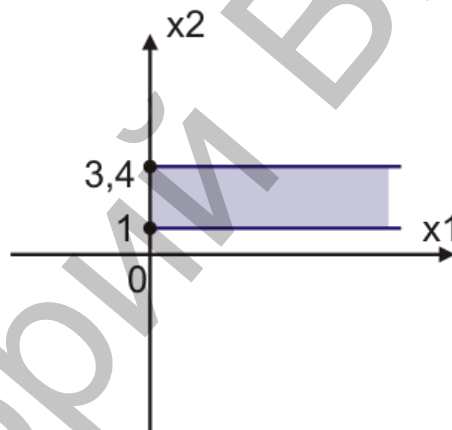
Рис. 2.4. Граничные условия.
